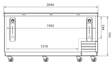
ВИД СПЕРЕДИ
